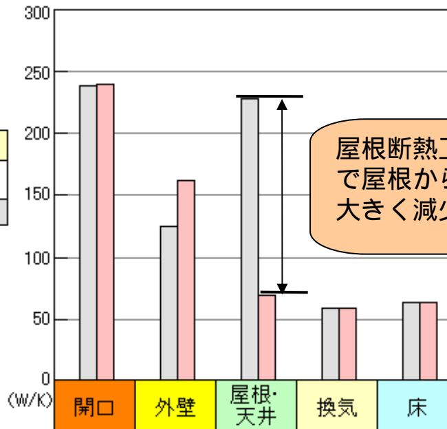
■(部位別)建物から損失する熱量(W/K)の比較
